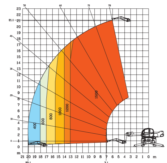
液压支腿完全伸出, 车身旋转 带 1500公斤吊臂
