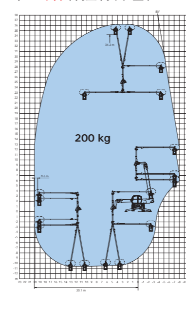
液压支腿完全伸出, 车身旋转 带 3D平台 (向上/向下位置)
